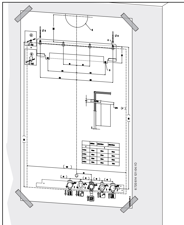
Рис. 6 монтажний шаблон
