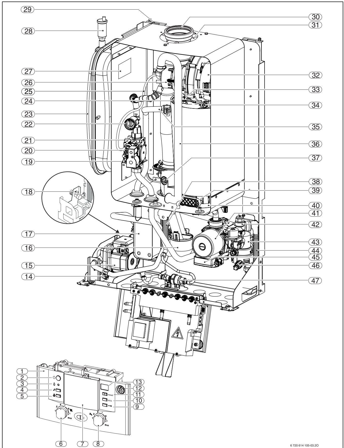
Рис. 3 Опалювальний прилад
