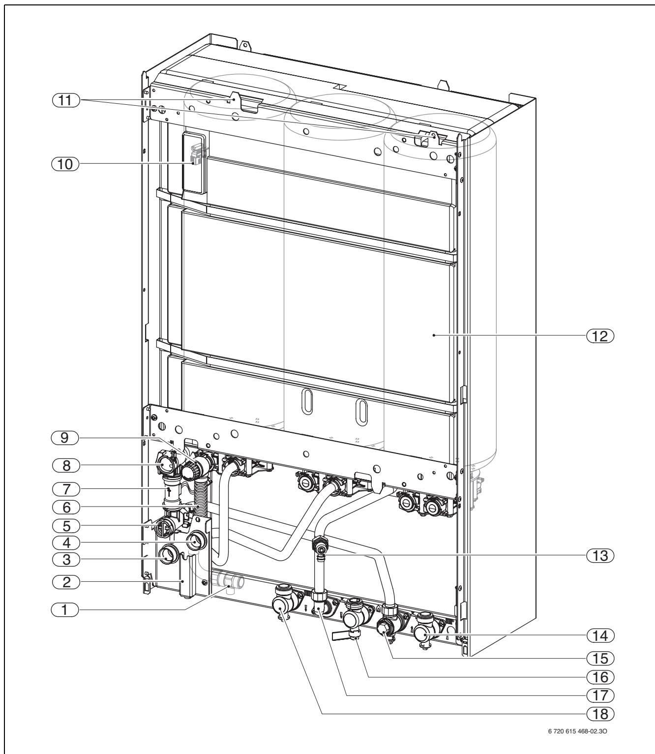
Рис. 4 Шаровий накопичувач
