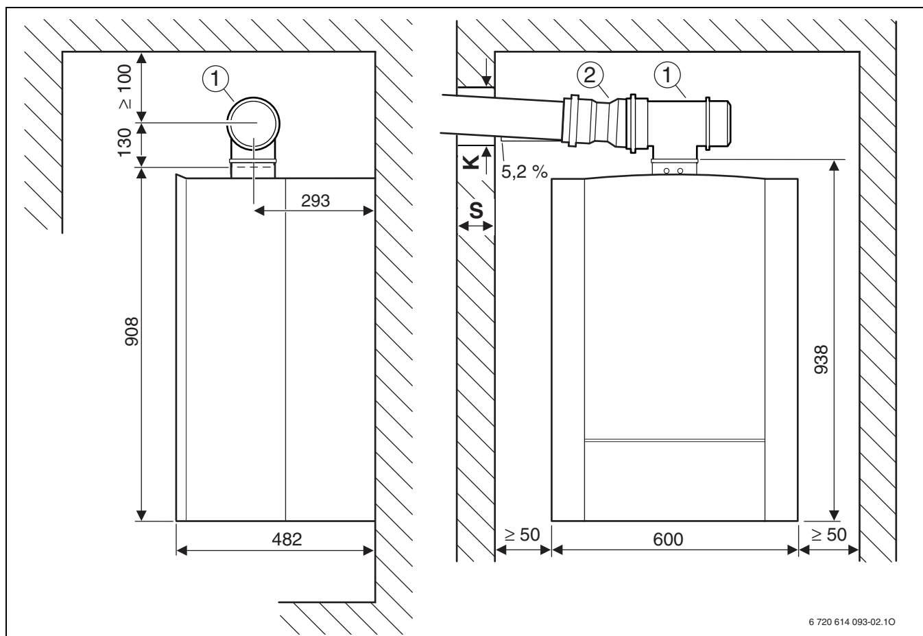
Рис. 6 Відвід димових газів Ø 60/100 мм
