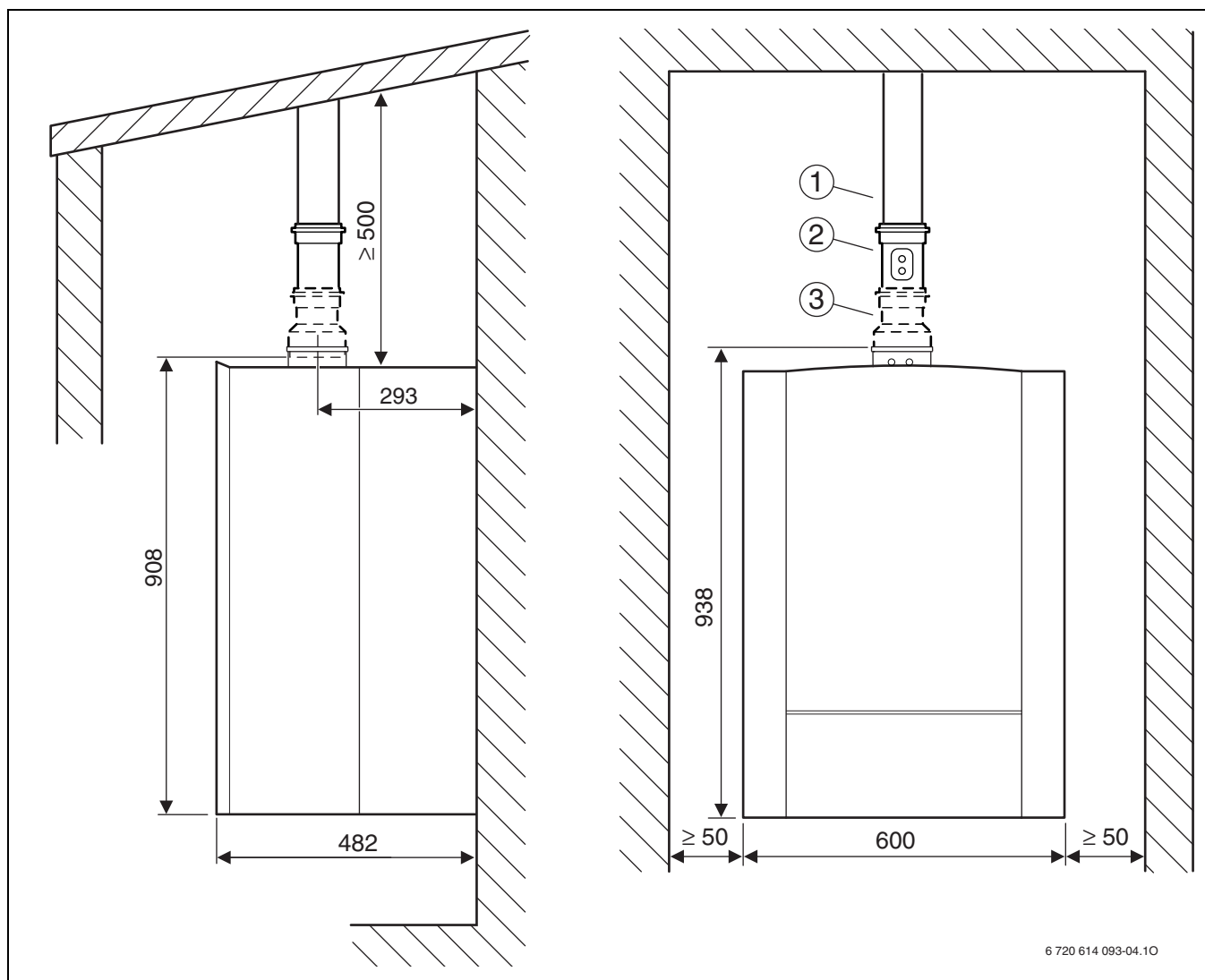
Рис. 8 Похилий дах
