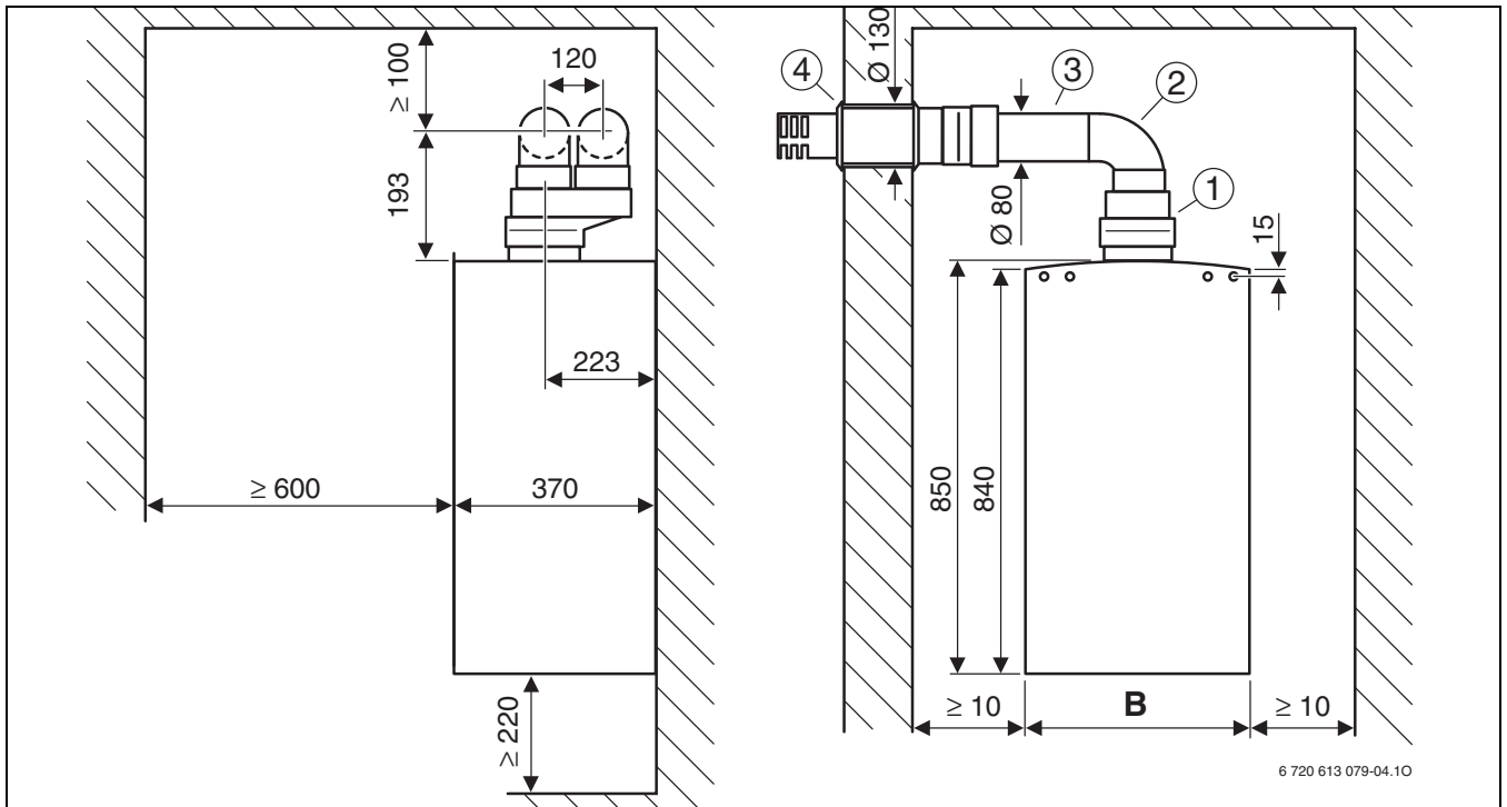
Рис. 9 Димовідвід по C 12
