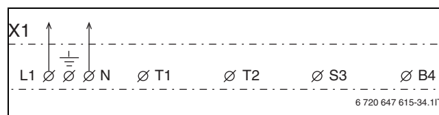
Мал. 31 Індикація Головного вимикача «Вимк.»
