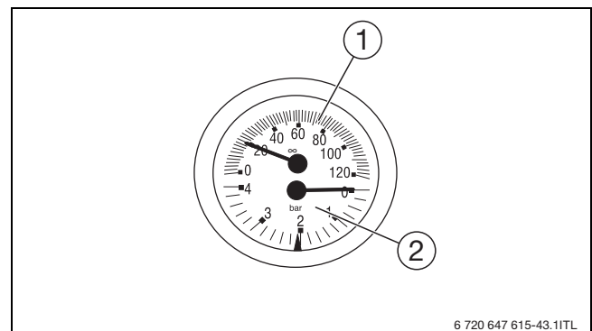
Мал. 4 Термометр/манометр
