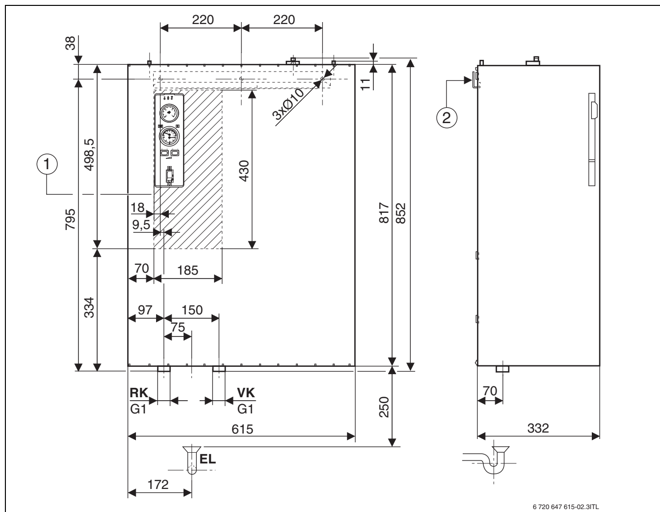
Мал. 3 Розміри та підключення Tronic 5000H 22—60
