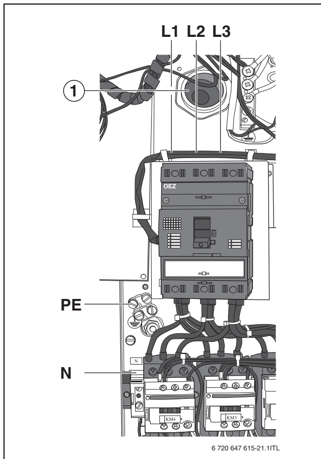
Мал. 8 Підключення до електромережі 36—60 кВт (5-проводова мережа)
