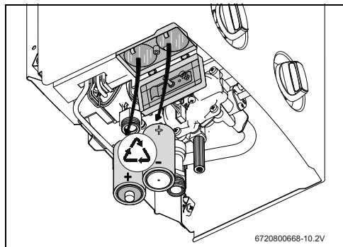
Мал. 5 Відсік для розміщення батарей
