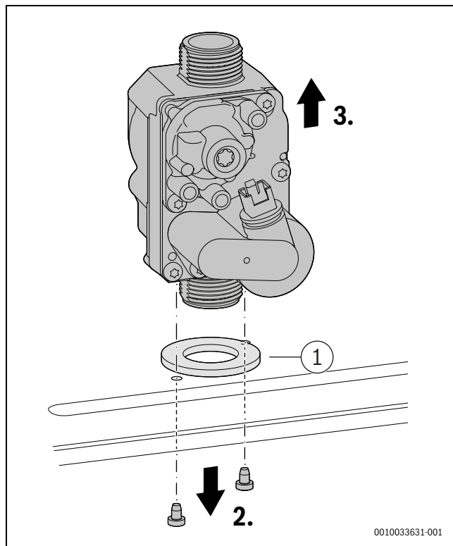
Мал. 135 Демонтаж газової арматури
