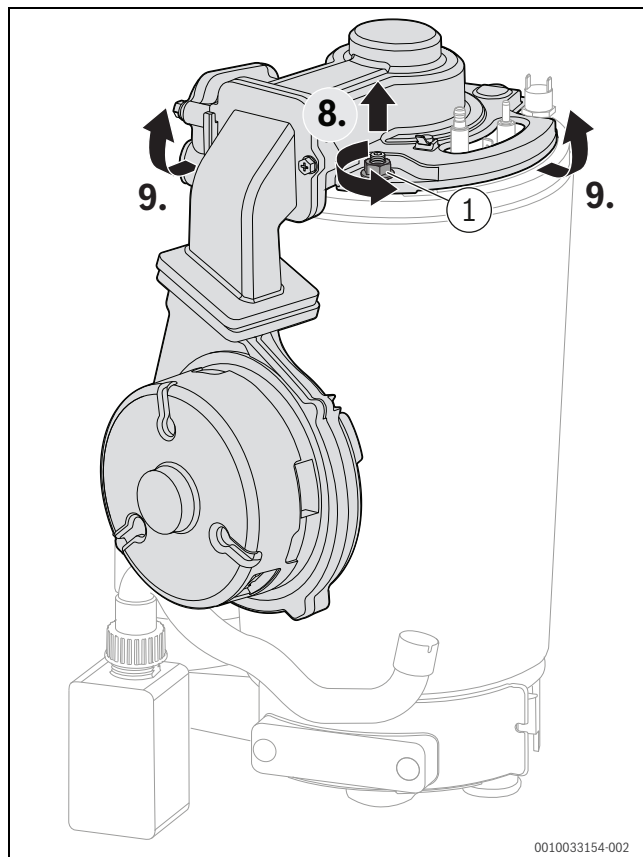
Мал. 114 Знімання кришки пальника разом з вентилятором та змішувальною камерою
