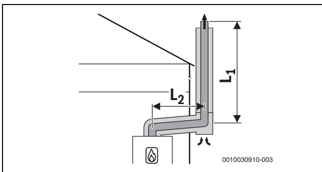
Мал. 28 Система подачі повітря для горіння та відпрацьованих газів у концентричних трубах згідно з C_{53x} на зовнішній стіні
