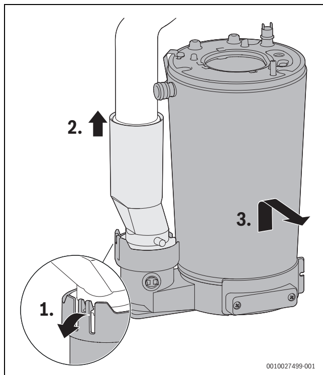
Мал. 127 Демонтаж котлового блока, який включає камеру згоряння і теплообмінник
