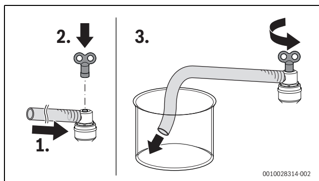
Мал. 71 Видалення повітря з контуру гарячої води та з опалювального контуру
