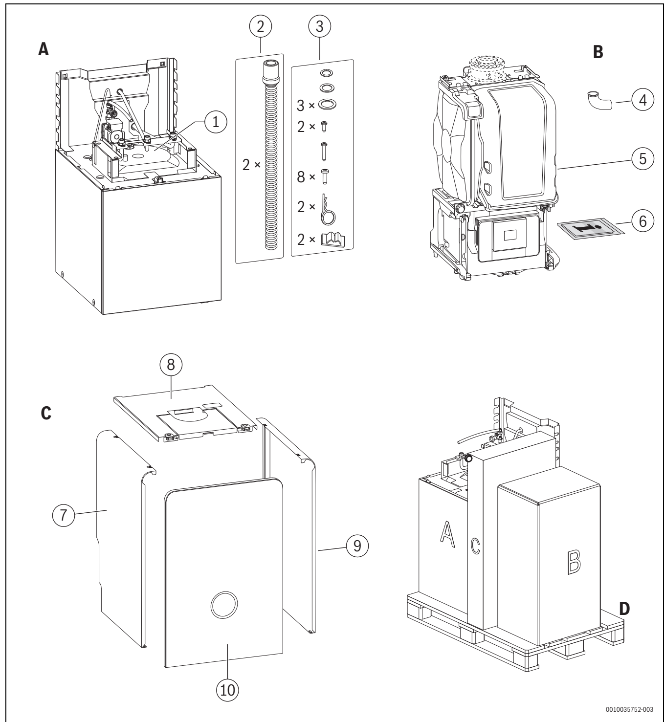
Мал. 4 Комплект поставки
