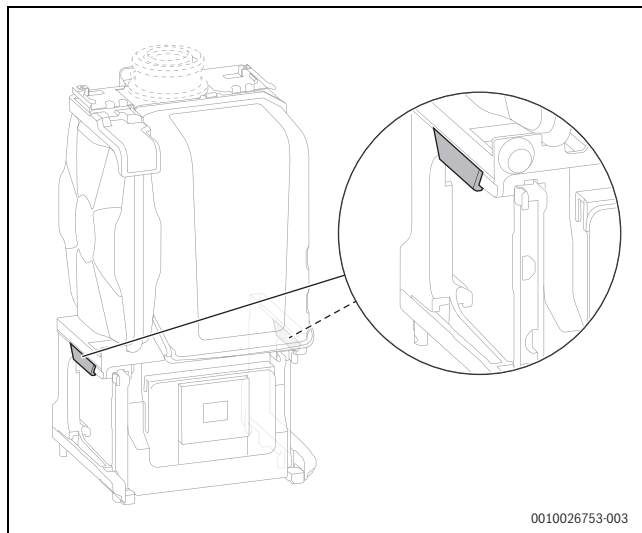
Мал. 50 Підніміть прилад за частини виділені сірим кольором та перевезіть до баку
