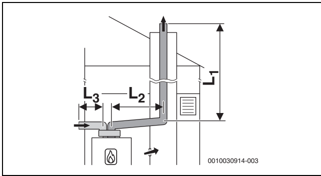
Мал. 27 Система відведення димових газів із жорсткою конструкцією відповідно до C_{53} у шахті та система транспортування повітря для горіння та відпрацьованих газів із окремими трубами для подачі повітря та трубопроводом для відведення димових газів у котельному приміщенні
