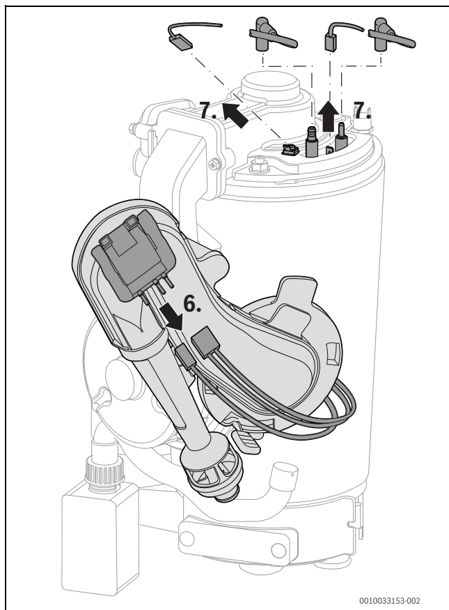
Мал. 113 Знімання кабелів
