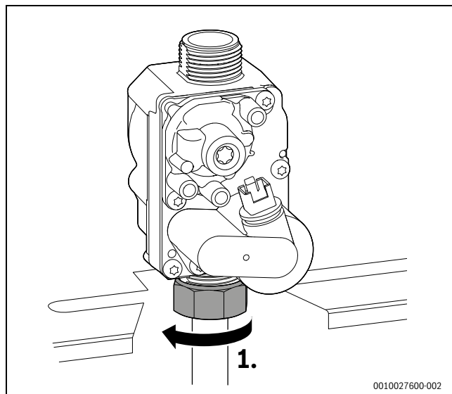
Мал. 134 Відкручування гайки
