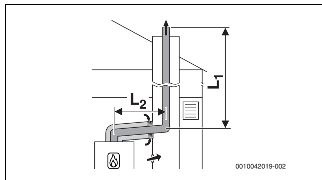
Мал. 31 Система відведення димових газів у шахті із жорсткою конструкцією відповідно до B 53p з подачею повітря з приміщення через концентричну систему транспортування повітря для горіння та відпрацьованих газів у котельному приміщенні
