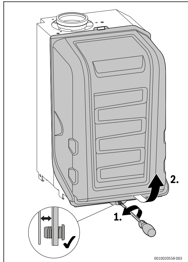
Мал. 97 Зніміть кришку пальника
