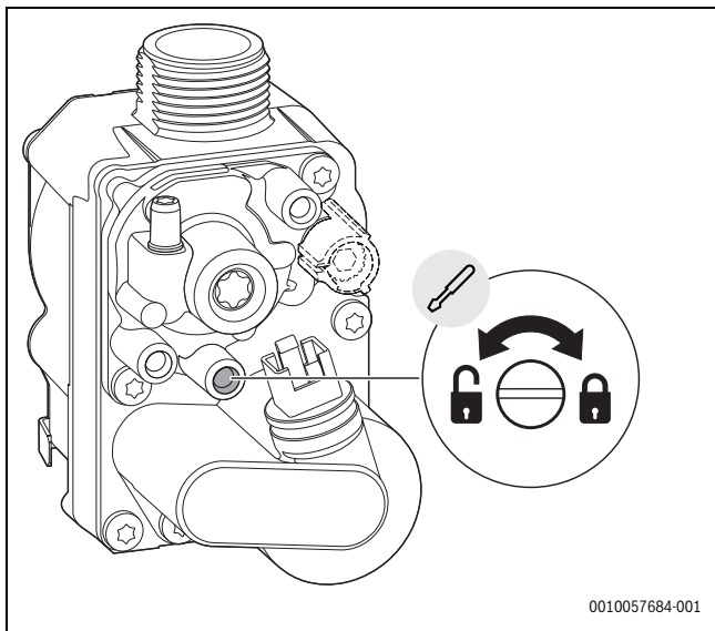
Мал. 98 Вимірювання тиску підключення газу
