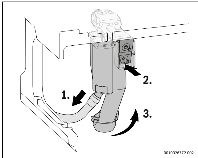
Мал. 141 Демонтаж сифона для конденсату
