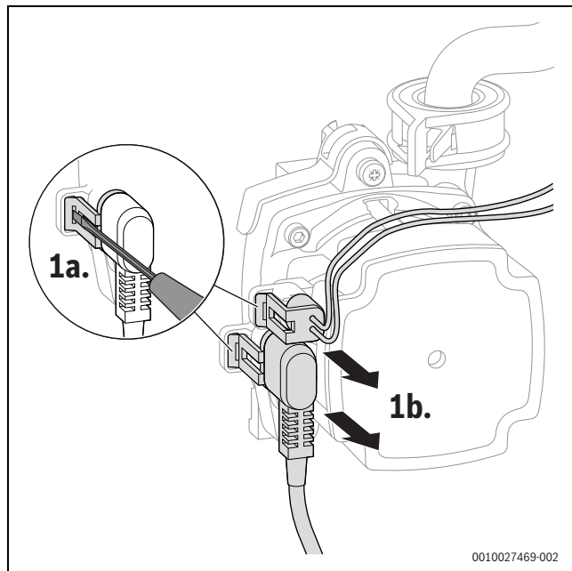
Мал. 128 Зніміть штекер з насоса опалювального контуру
