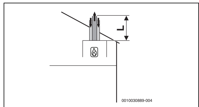
Мал. 24 Вертикальна концентрична система транспортування повітря для горіння та відпрацьованих газів згідно з C 33x
