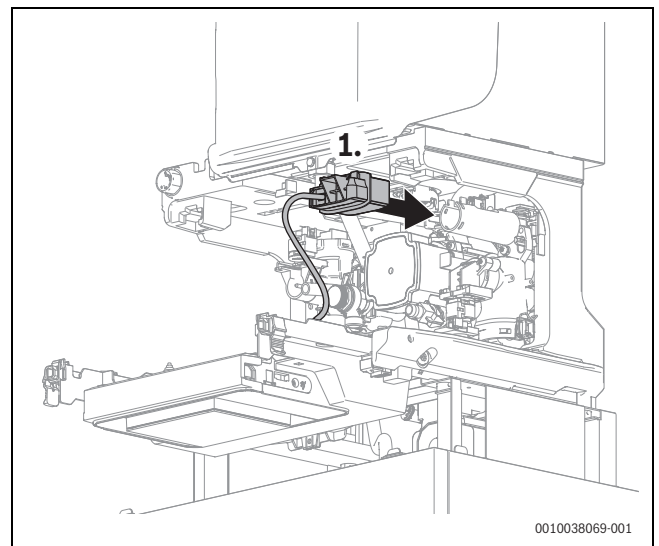
Мал. 58 Спрямуйте тримач Кей до задньої частини пристрою
