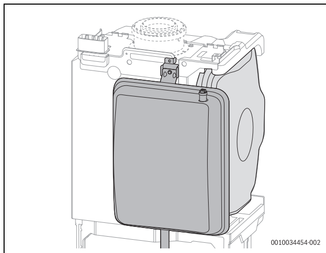
Мал. 40 На приладі встановлено 2 мембранні компенсаційні баки
