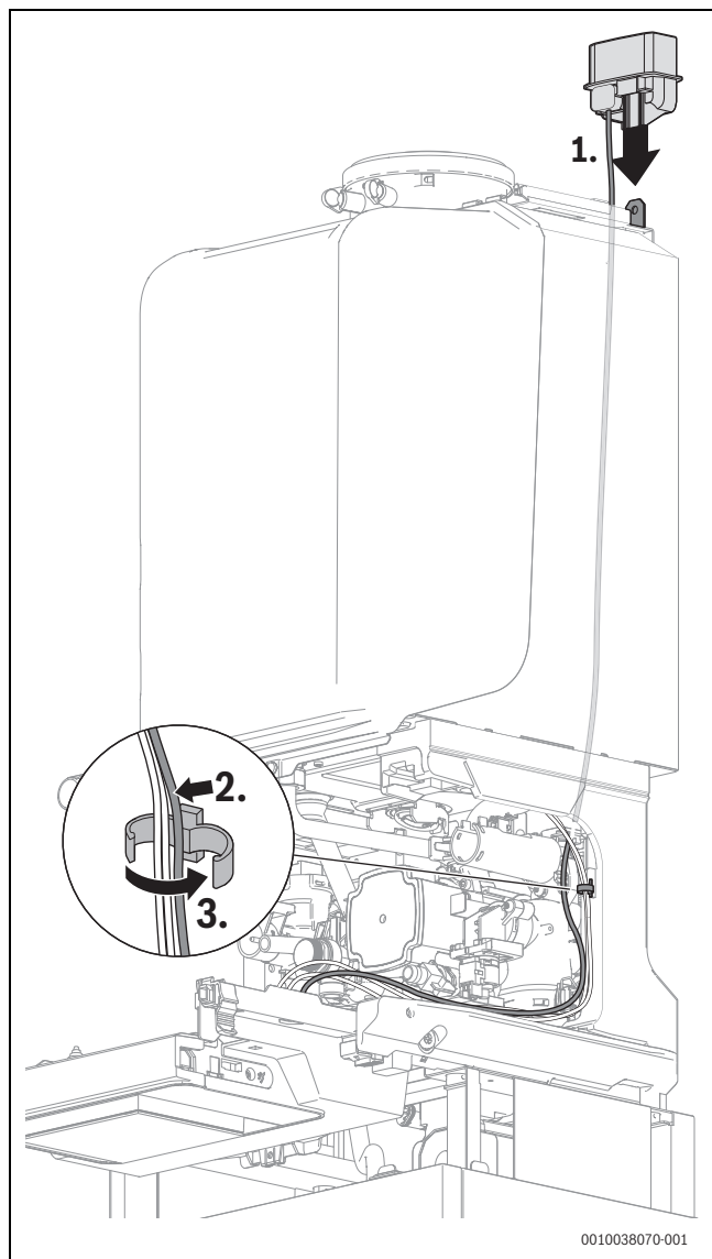
Мал. 59 Вставте тримач Keu у роз'єм та зафіксуйте кабель тримачем кабелю
