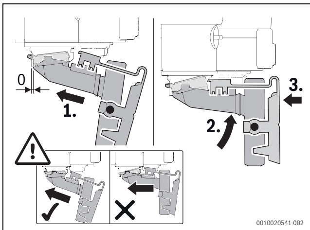
Мал. 144 Встановлення сифону для відведення конденсату
