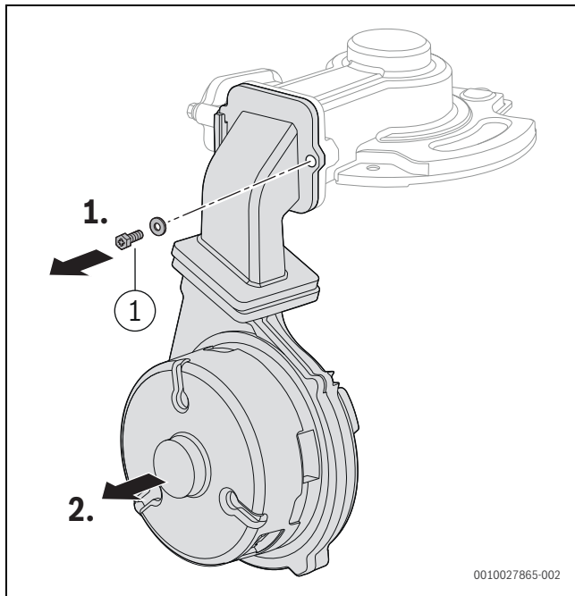
Мал. 115 Демонтаж вентилятора зі змішувальною камерою
