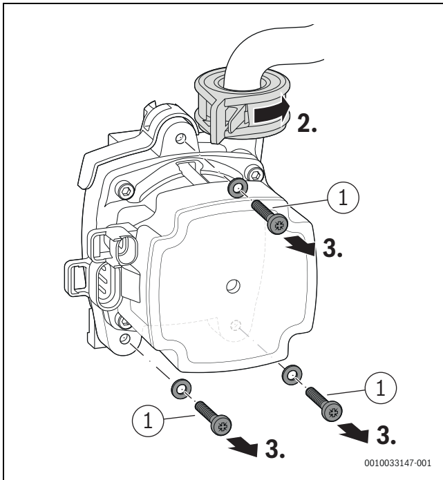
Мал. 129 Розблокуйте насос опалювального контуру та зніміть гвинти
