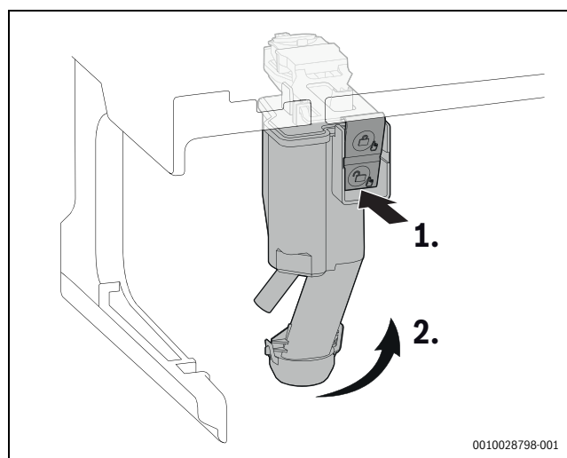
Мал. 53 Витягніть сифон для відведення конденсату
