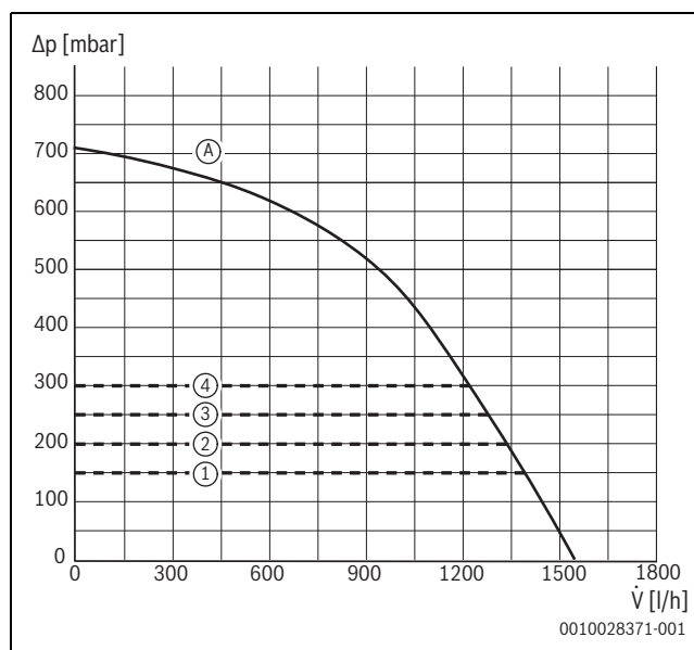
Мал. 150 Характеристики насоса і крива характеристик насоса (17/24 kW)
