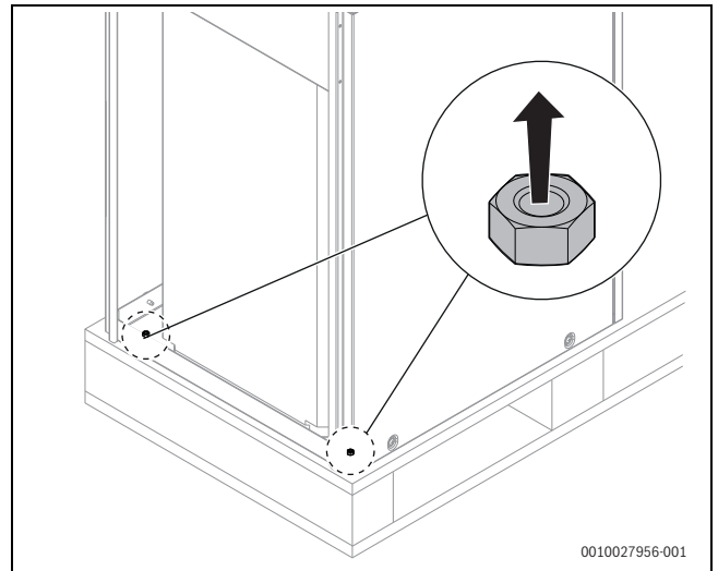
Мал. 43 Зніміть нижній транспортувальний запобіжник на зворотній стороні баку
