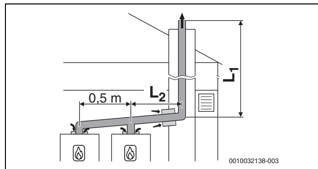
Мал. 34 Каскад з 2 приладами:
