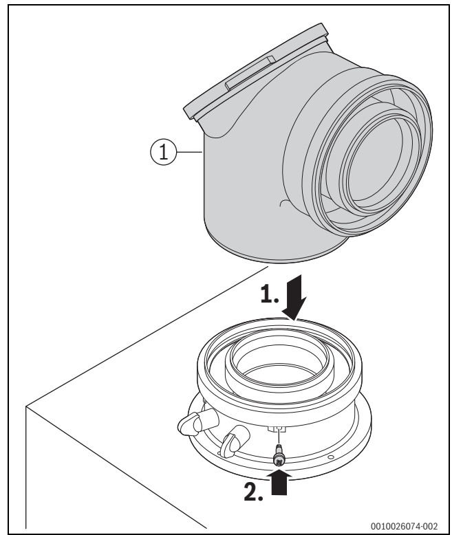
Мал. 66 Встановіть аксесуари для відведення відпрацьованих газів та зафіксуйте гвинтом
