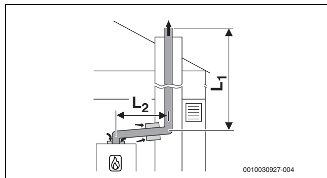
Мал. 30 Система відведення димових газів у шахті жорсткої конструкції відповідно до B 53p з подачею повітря у прилад з приміщення та концентричною з'єднувальною деталлю між котельним приміщенням та шахтою
