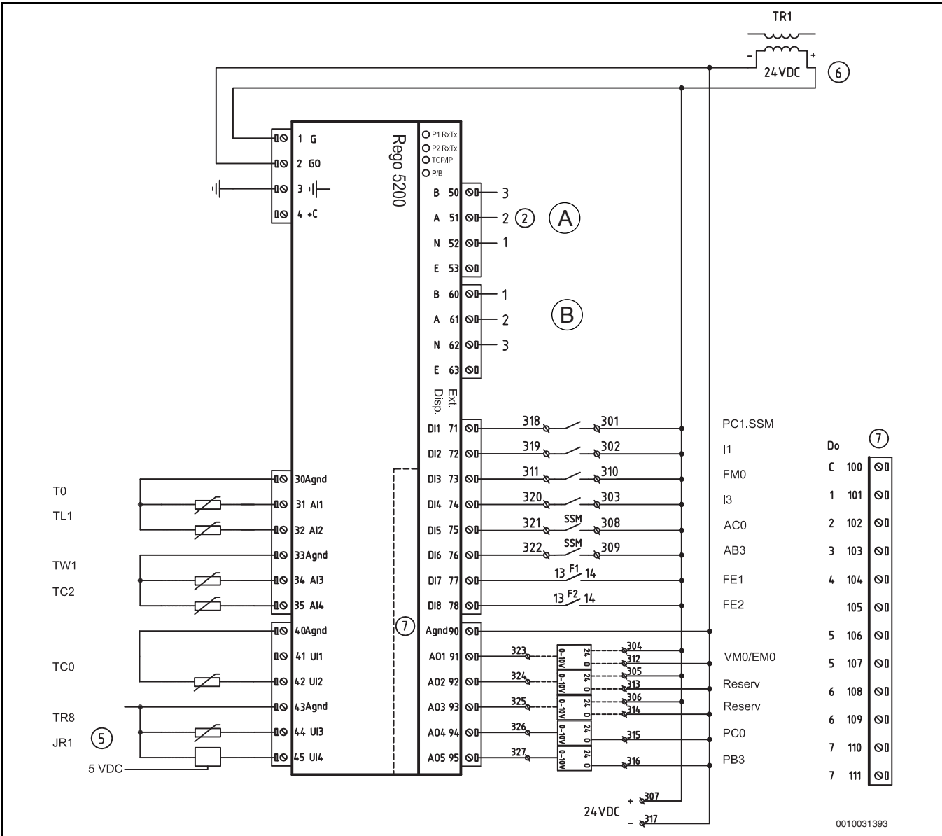
Мал. 27 Схема електричних з'єднань із запобіжником системи керування
