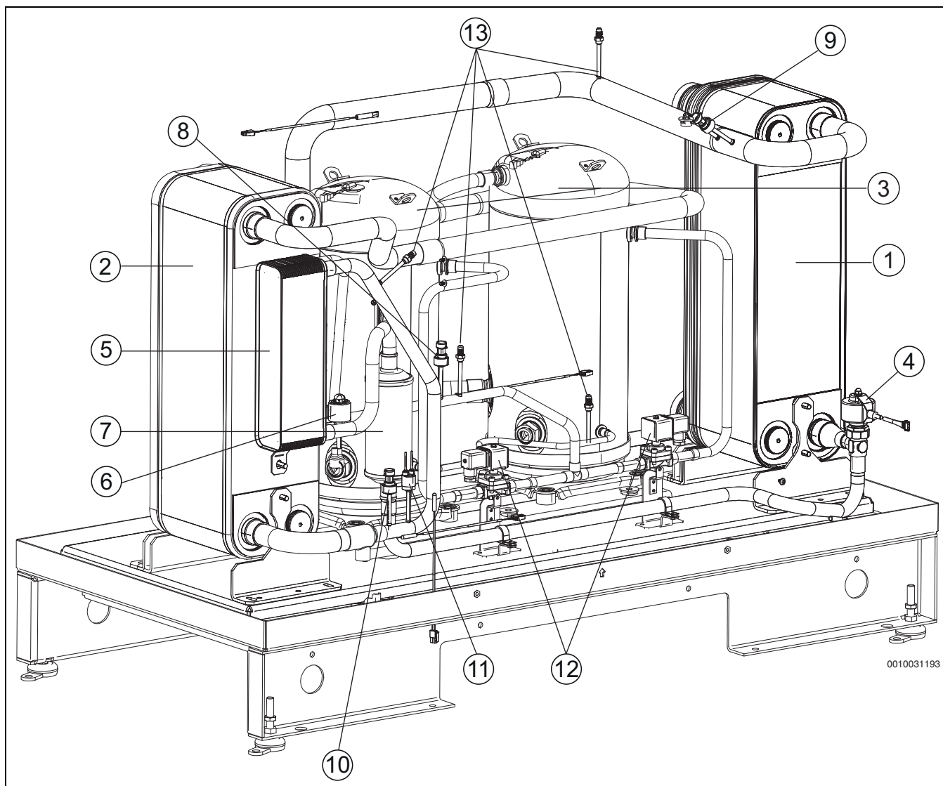
Мал. 2 Огляд виробу
