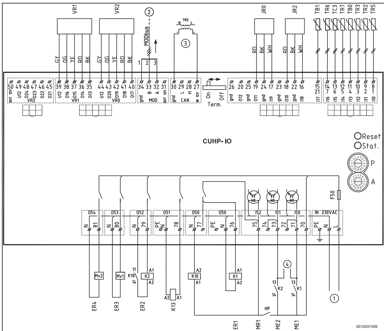
Мал. 28 Схема електричних з'єднань, тепловий насос із контактором
