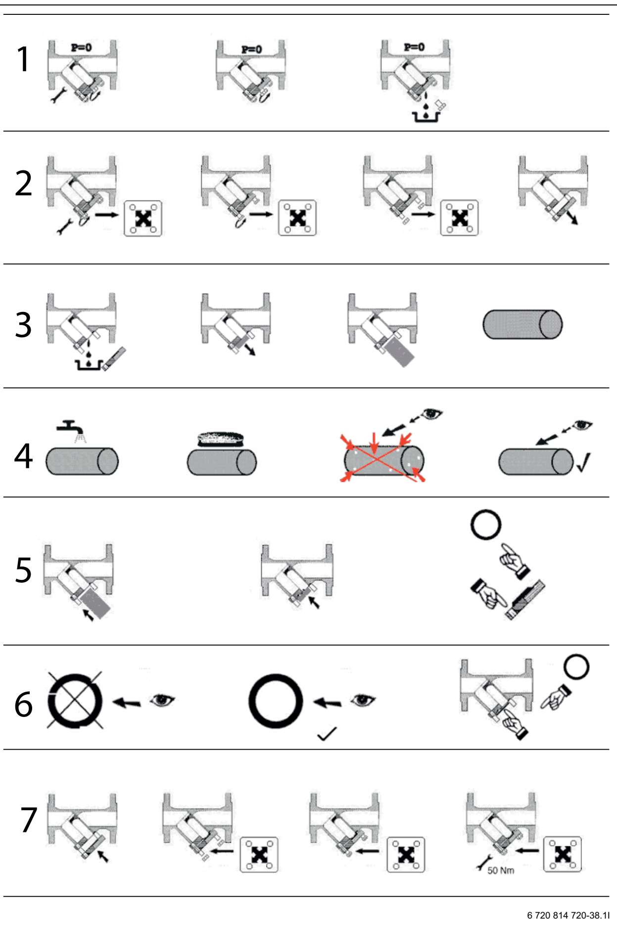
Мал. 17 Очищення фільтрувальної решітки у фланцевому фільтрі
