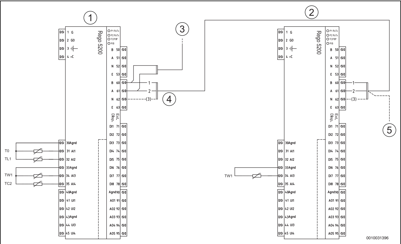
Мал. 33 Схема електричних з'єднань, послідовне з'єднання
