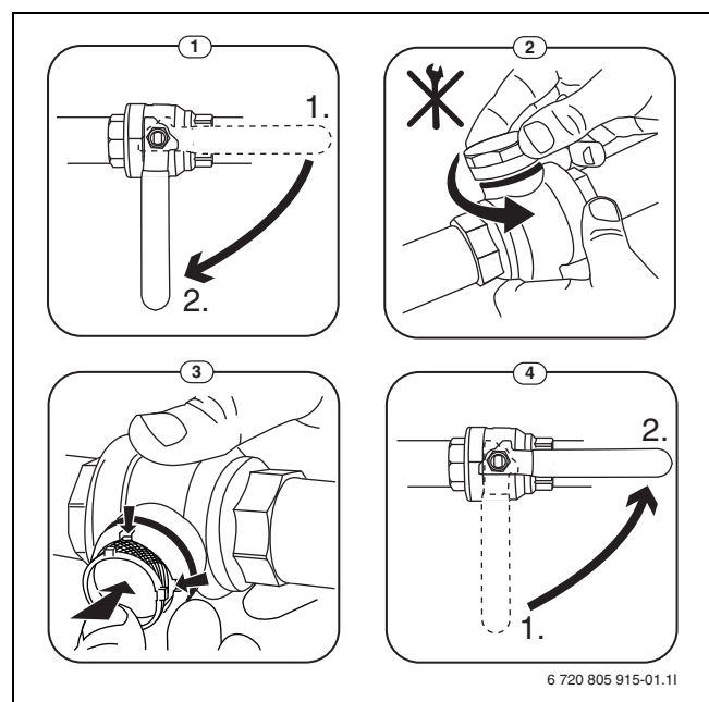
Мал. 15 Очищення фільтрувальної решітки
