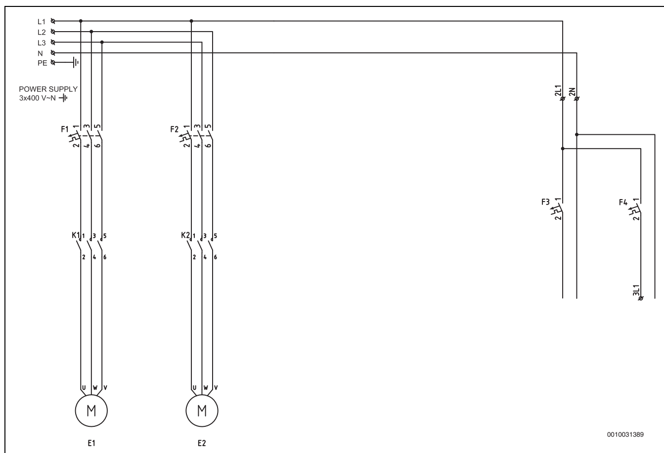
Мал. 24 Схема електричних з'єднань, підключення до електромережі з контактором
