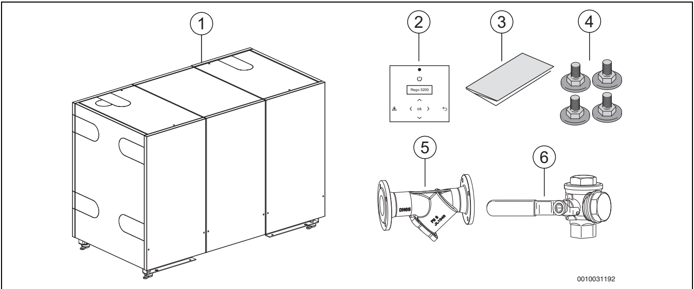
Мал. 1 Стандартна поставка
