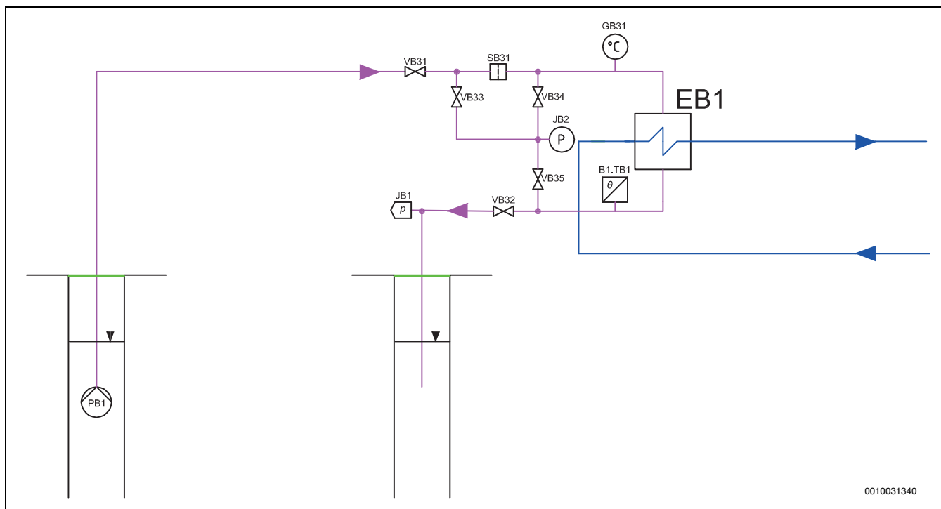
Мал. 38 Система ґрунтової води
