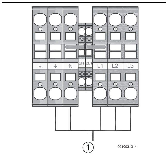
Мал. 20 Подача напруги живлення в стандартному виконанні
