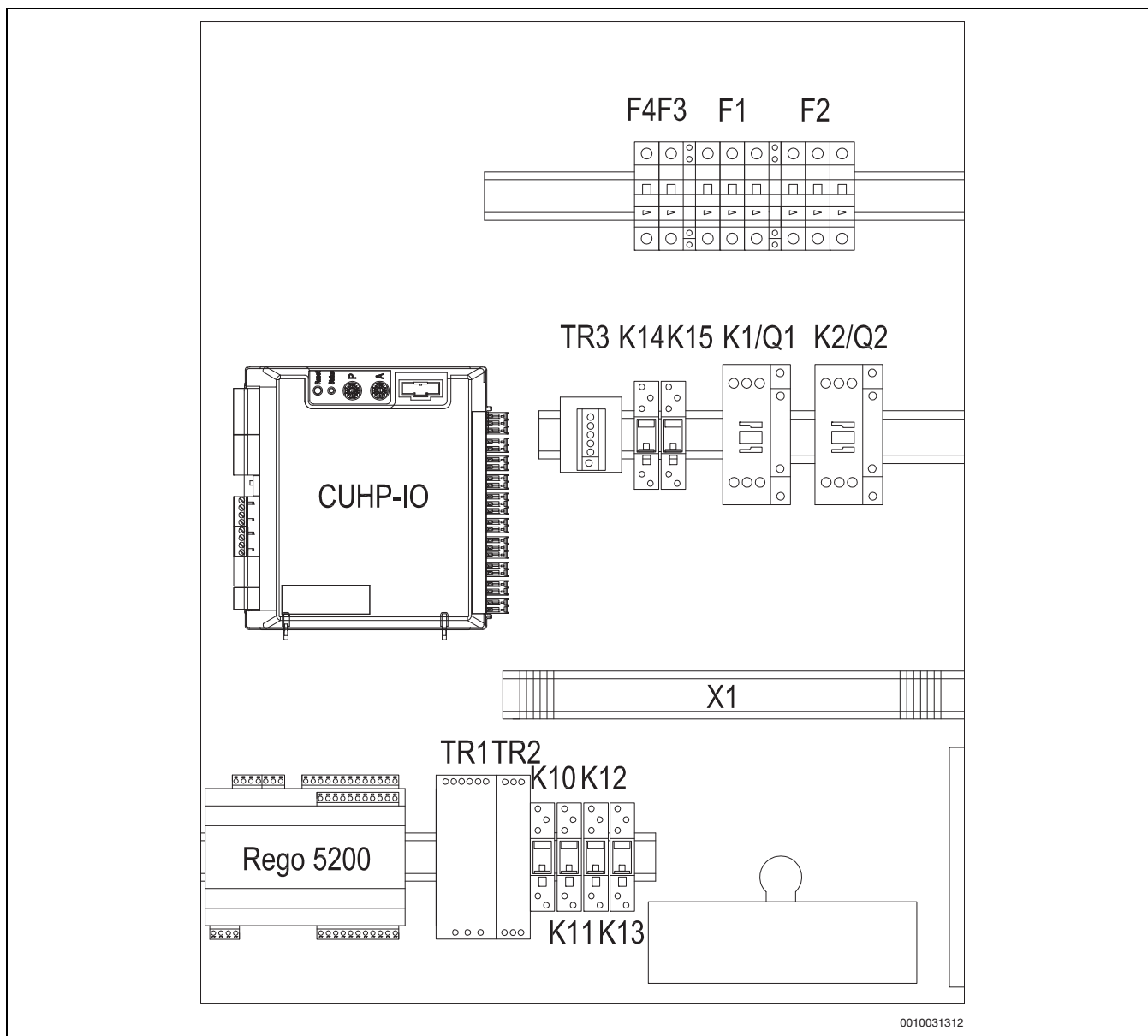
Мал. 18 Огляд електричного модуля
