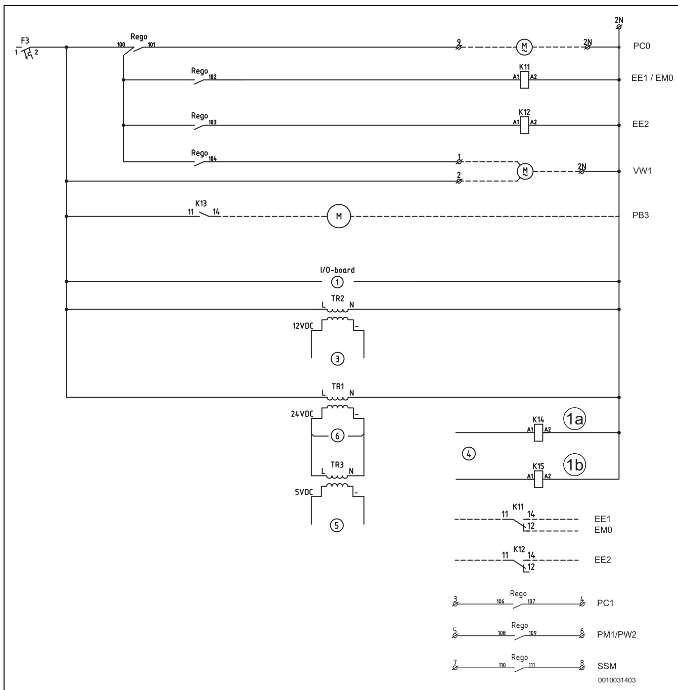
Мал. 30 Схема електричних з'єднань, тепловий насос
