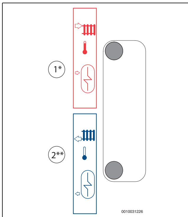
Мал. 11 Підключення теплового насоса до системи опалення
