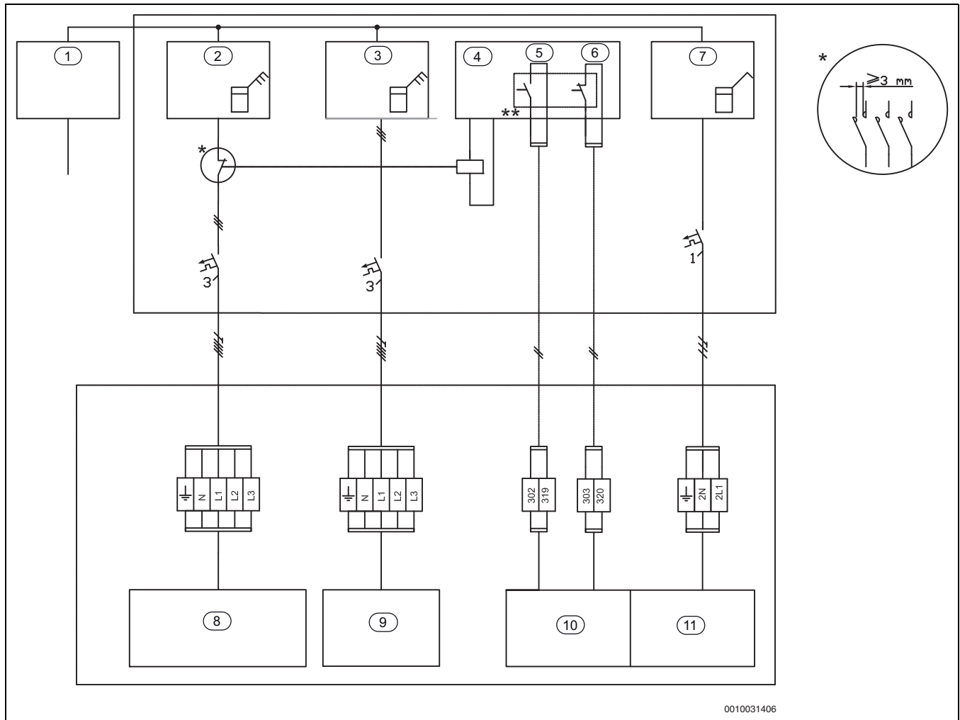
Мал. 36 EVU, тип 2 із вимкненням компресора
