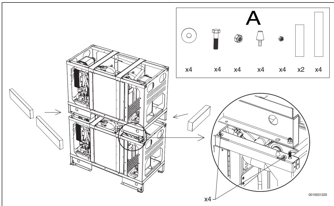
Мал. 9 Встановлення двох теплових насосів у колону
