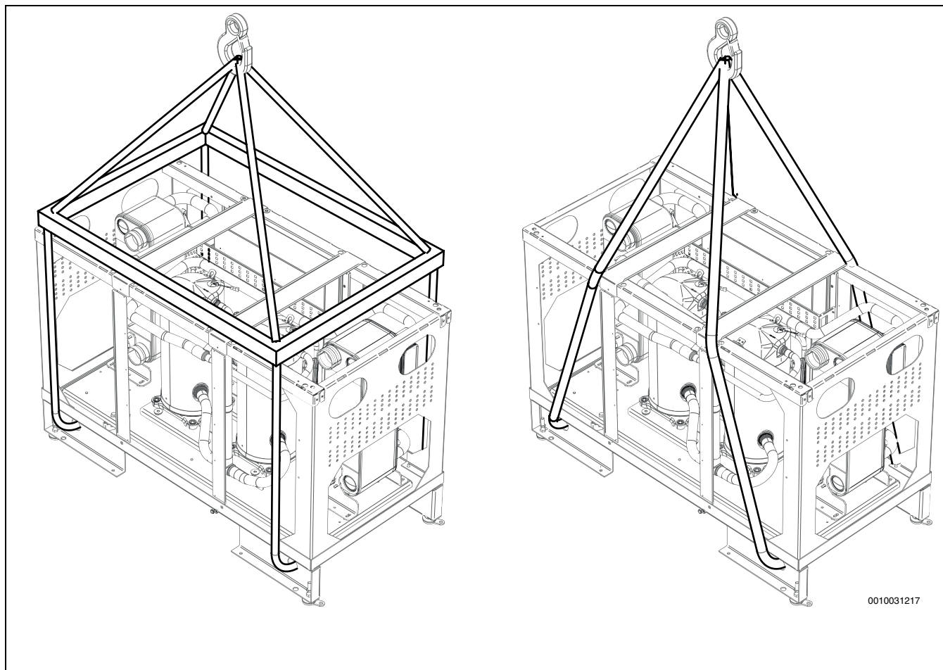
Мал. 8 Варіанти транспортування теплового насоса 22–48 кВт
