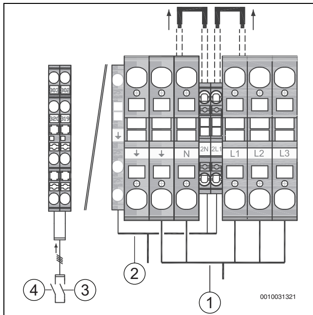
Мал. 21 Подача напруги живлення за схемою низького тарифу
