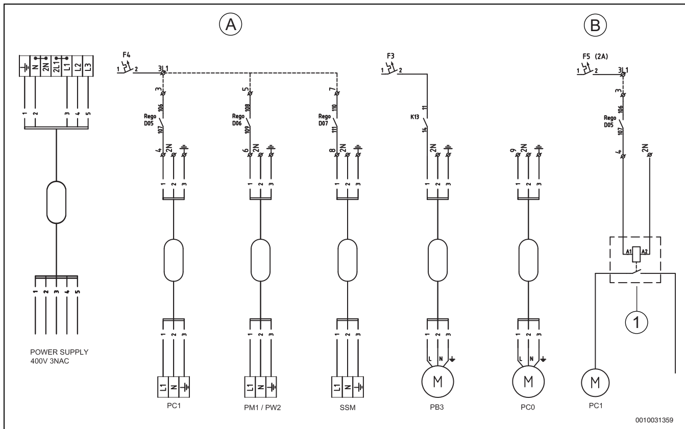
Мал. 22 Схема зовнішніх з'єднань
