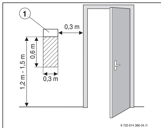
Мал. 12 Рекомендоване положення встановлення датчика кімнатної температури
