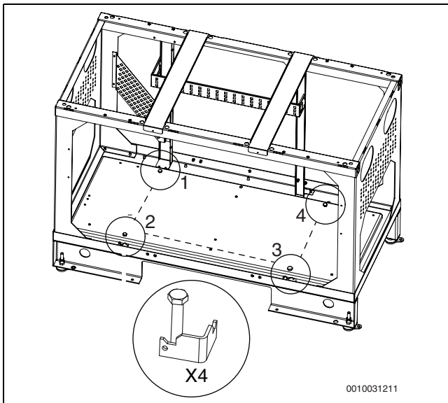
Мал. 6 Захист під час транспортування, тепловий насос
