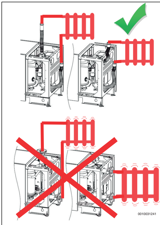
Мал. 14 Зменшення вібрації в місцях з'єднання трубопроводу з системою опалення
