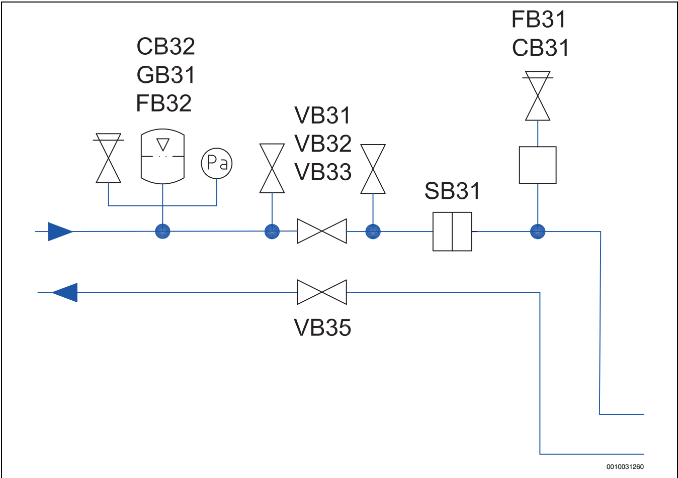
Мал. 16 Контур джерела з клапанами
