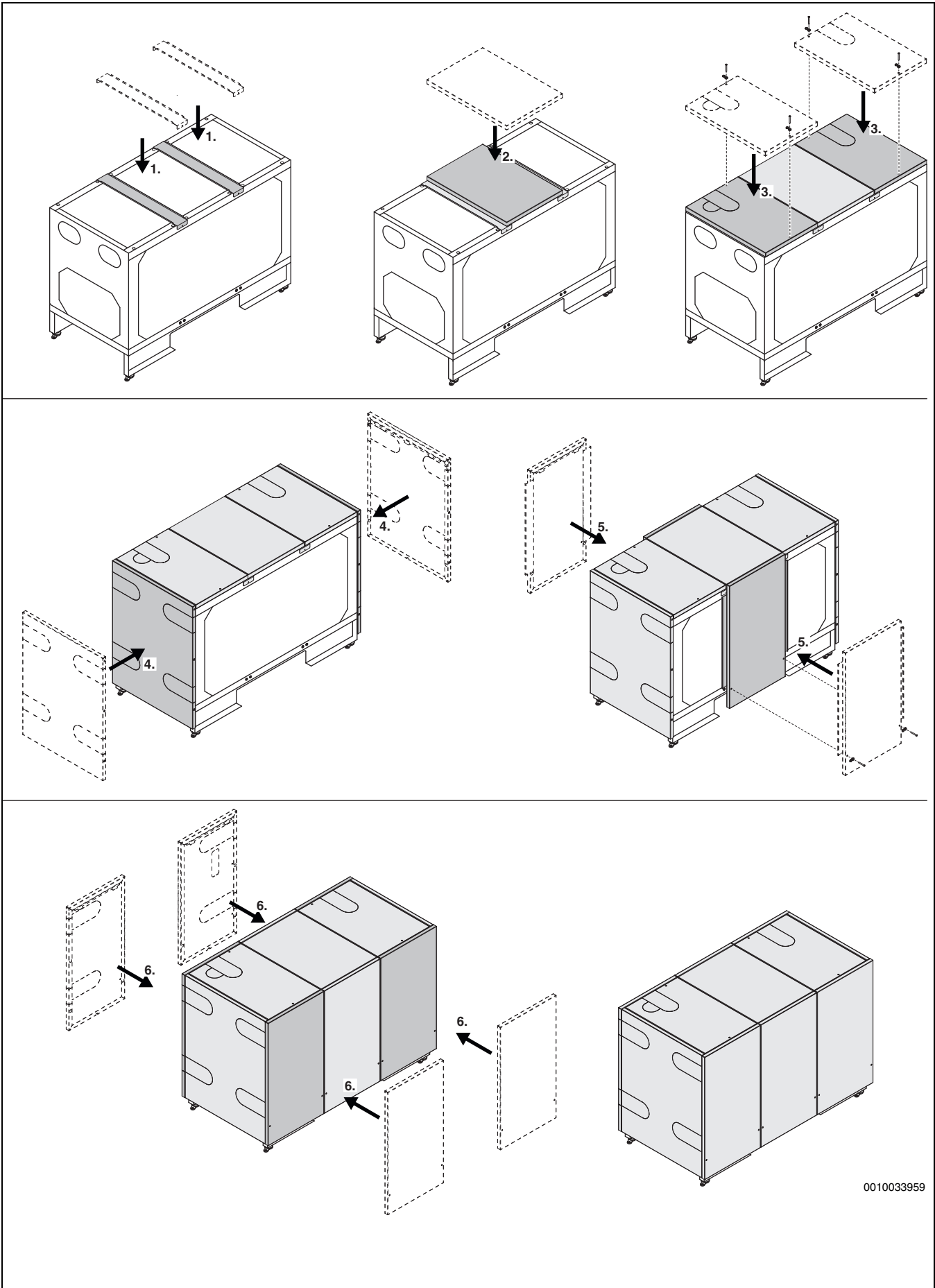
Мал. 13 Монтаж кришок
