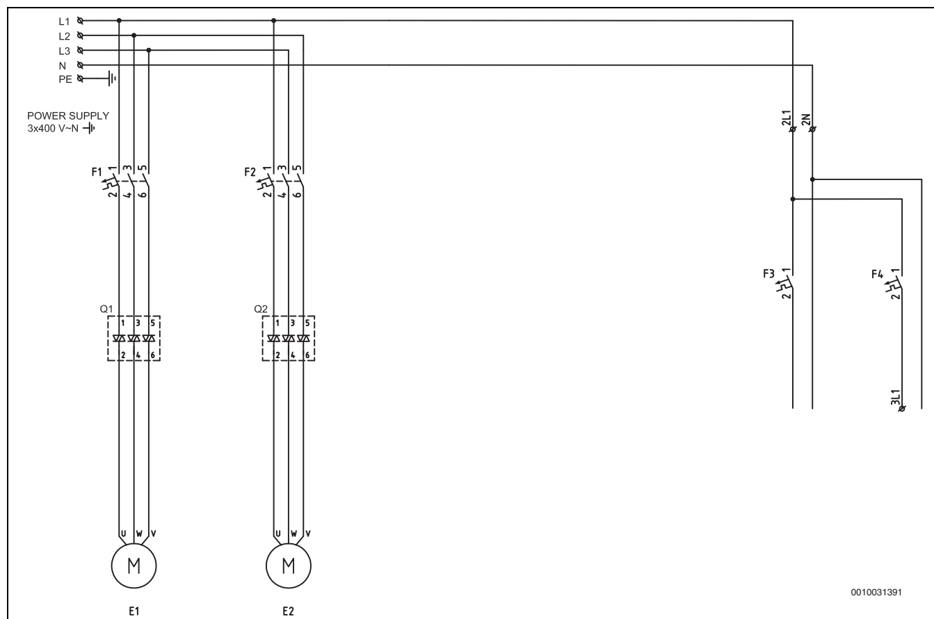
Мал. 25 Схема електричних з'єднань, підключення до електромережі, обмежувач пускового струму
