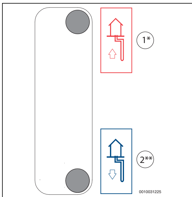
Мал. 10 Підключення теплового насоса до розсільного контуру
