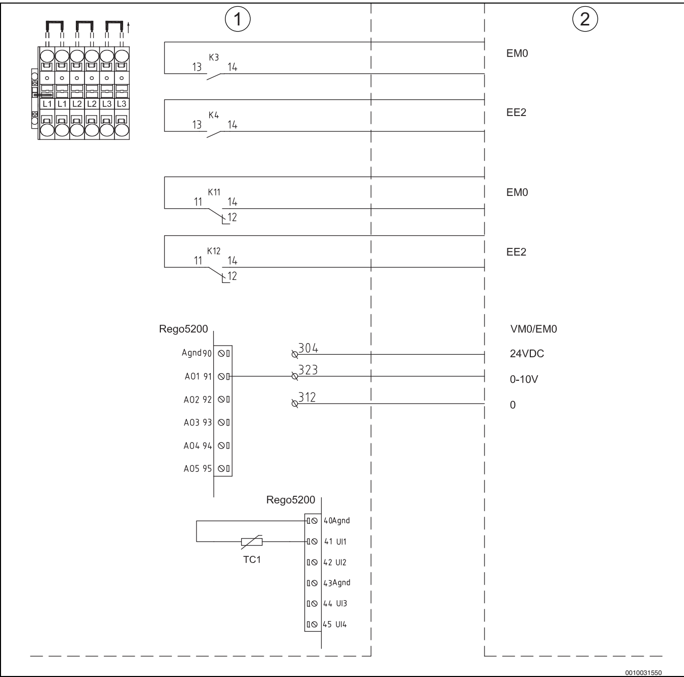
Мал. 31 Підключення зовнішнього шунтованого додаткового джерела тепла 22–80 кВт
