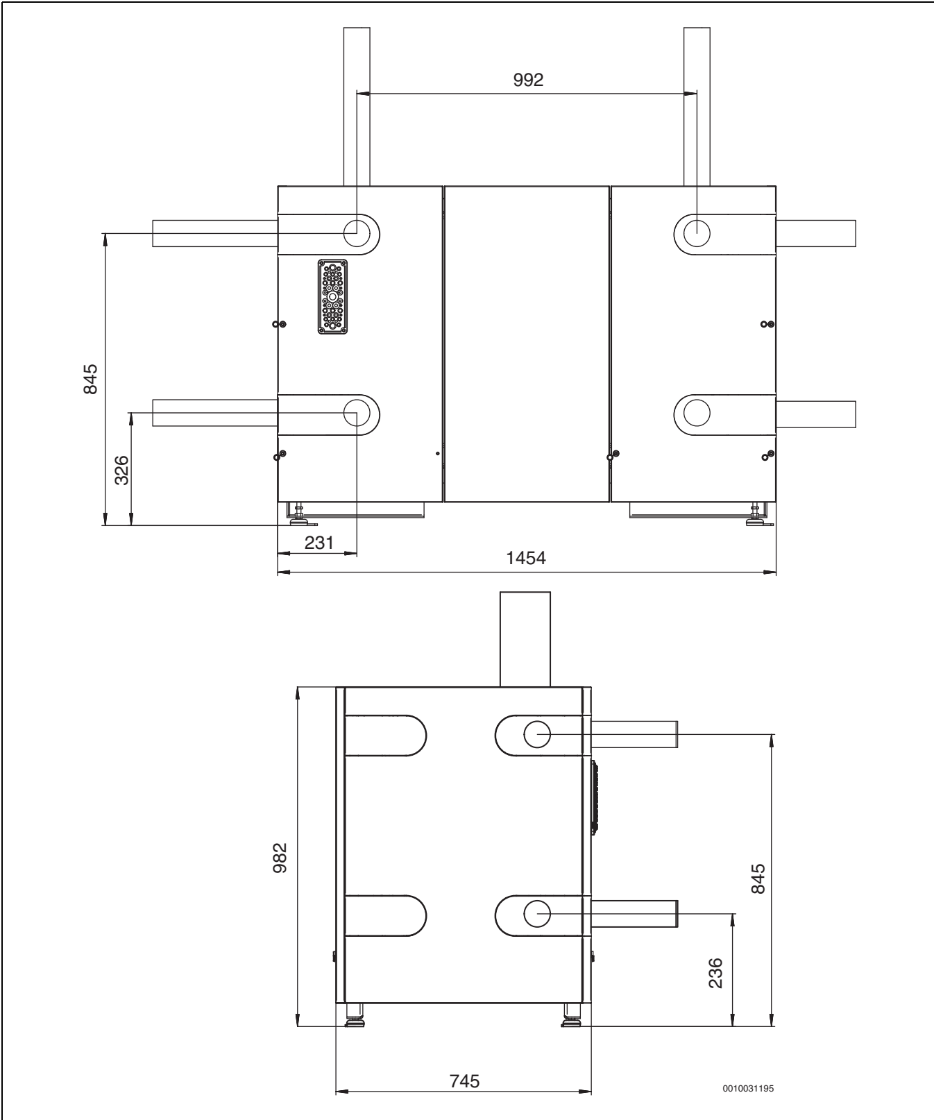
Мал. 3 Розміри теплового насоса
