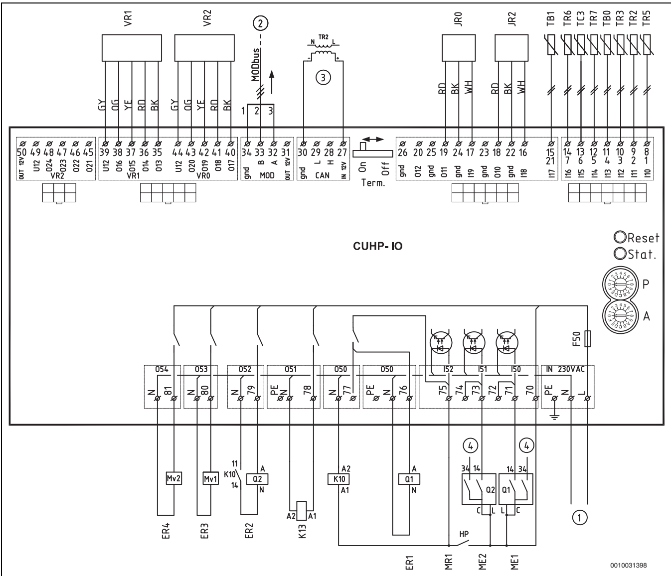
Мал. 29 Схема електричних з'єднань, тепловий насос з обмежувачем пускового струму
