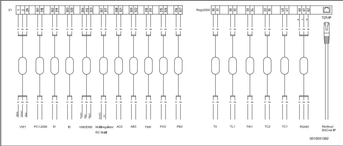
Мал. 23 Схема зовнішніх з'єднань
