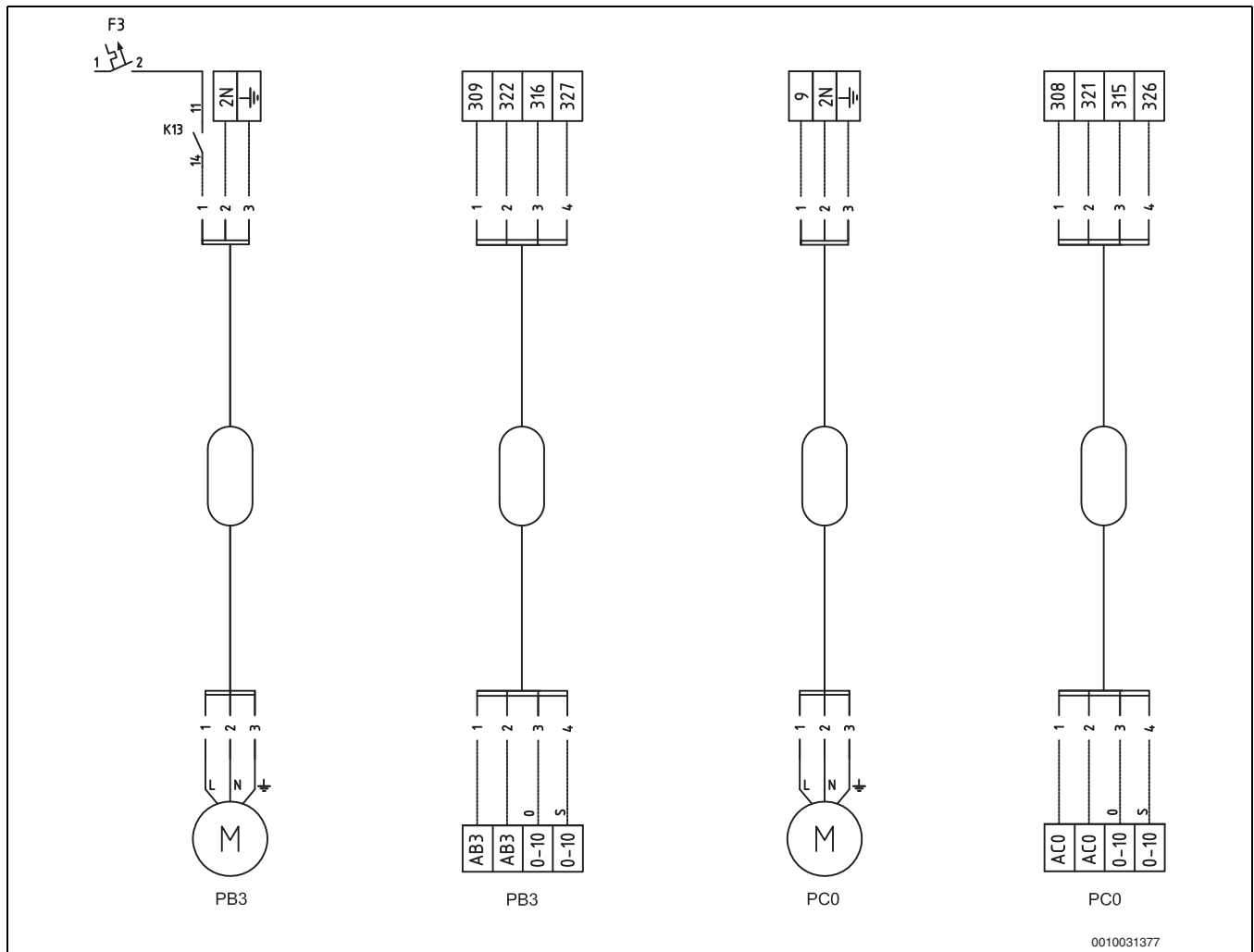
Мал. 32 Підключення насоса розсільного контуру/насоса опалювального контуру
