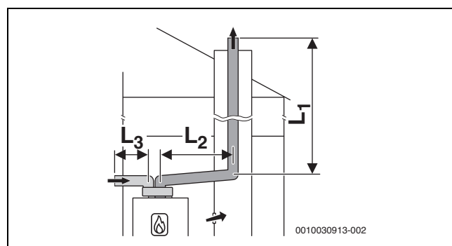
Мал. 13 Система відведення димових газів із жорсткою конструкцією відповідно до C_{53} у шахті та система транспортування повітря для горіння та відпрацьованих газів із окремими трубами для подачі повітря та трубопроводом для відведення димових газів у котельному приміщенні
