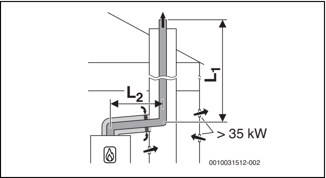
Мал. 17 Система відведення димових газів у шахті із жорсткою конструкцією відповідно до B_{33} з подачею повітря з приміщення через концентричну систему транспортування повітря для горіння та відпрацьованих газів у котельному приміщенні
