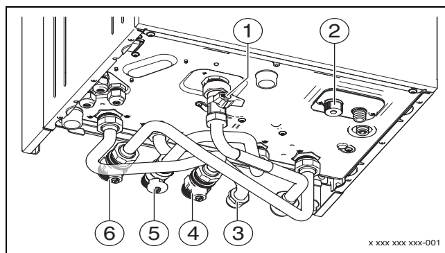
Мал. 30 Під'єднання трубопроводів з боку подачі газу та води xDOS GA 7
