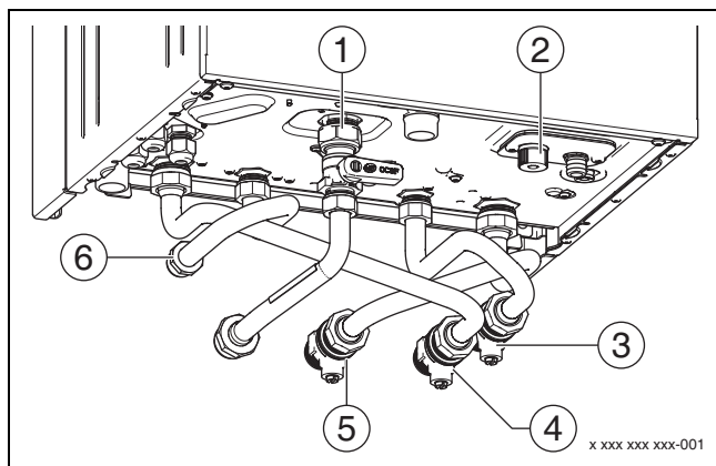
Мал. 29 Під'єднання трубопроводів з боку подачі газу та води xDOS GA 6
