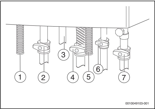
Мал. 27 Під'єднання з боку газо- та водопроводу (додаткова опція)
