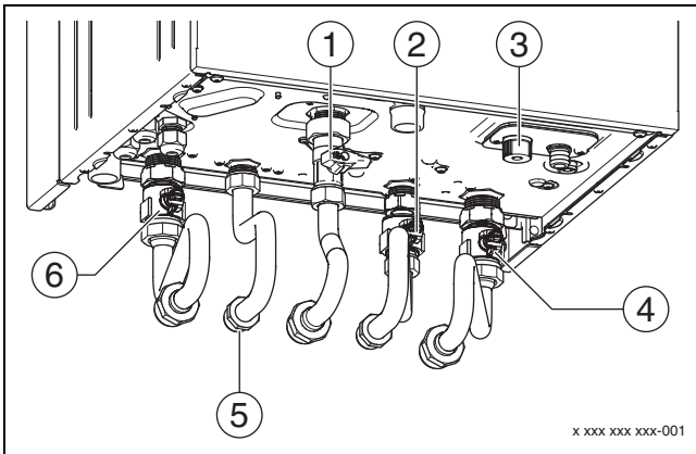
Мал. 33 Під'єднання трубопроводів з боку подачі газу та води xDOS GA 18
