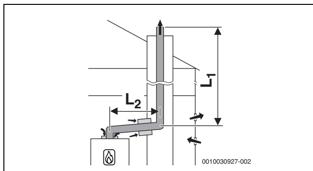
Мал. 16 Система відведення димових газів у шахті жорсткої конструкції відповідно до В 53p з подачею повітря у прилад з приміщення та концентричною з'єднувальною деталлю між котельним приміщенням та шахтою
