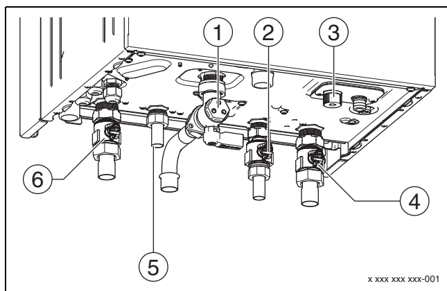
Мал. 28 Під'єднання трубопроводів подачі газу та води xDOS GA 5/ xDOS GA 15
