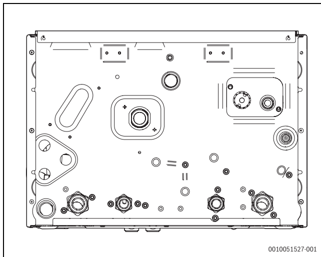
Мал. 35 Отвори для кабелів
