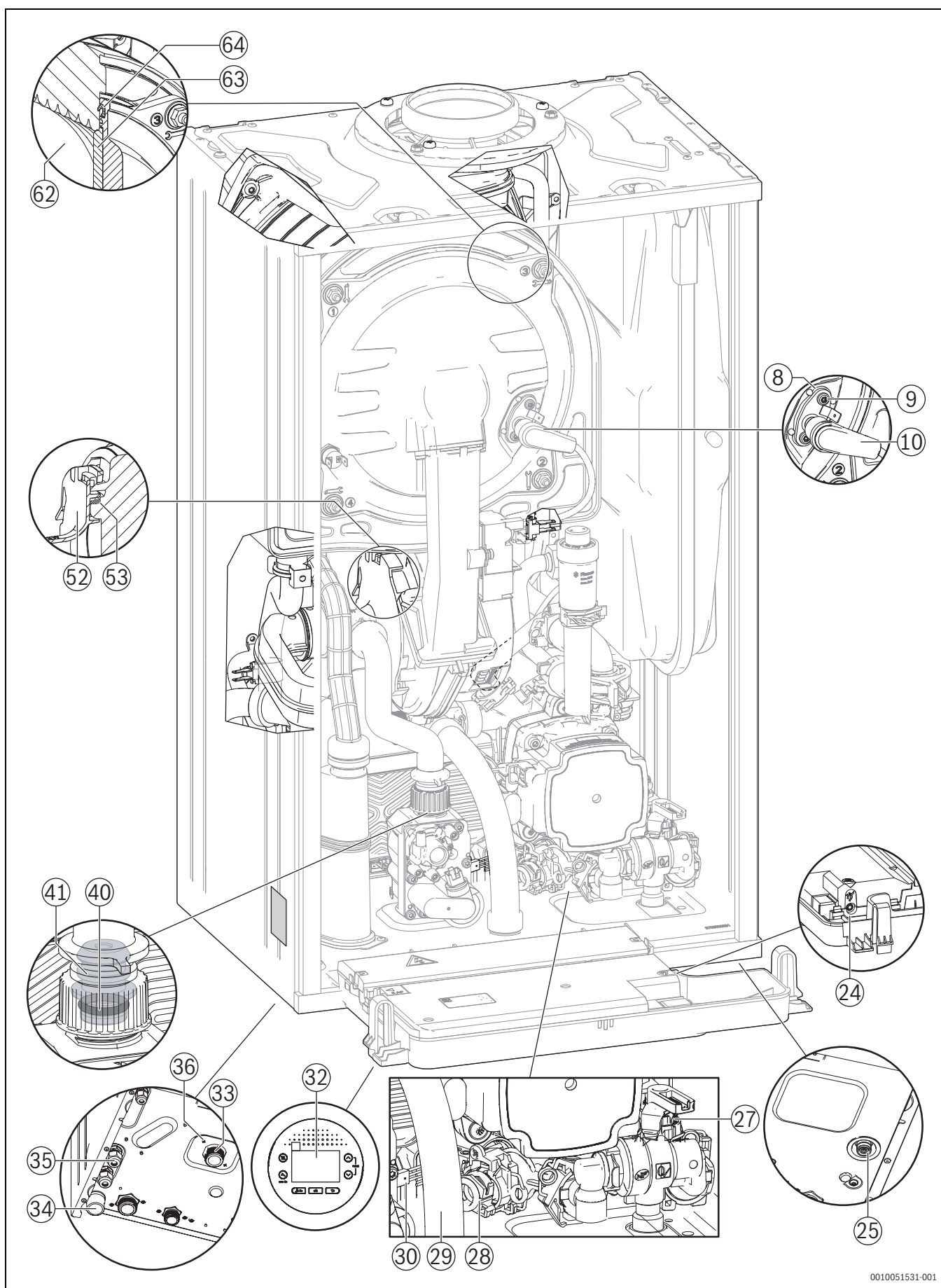
Мал. 4 Огляд виробу
