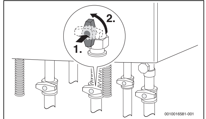
Мал. 3 Відкривання газового крана
