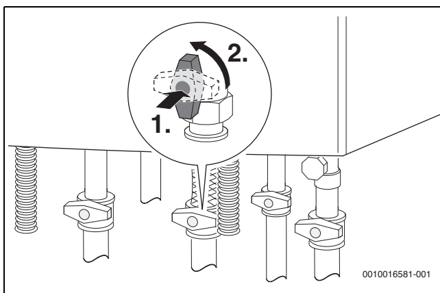
Мал. 5 Відкриття газового крана
